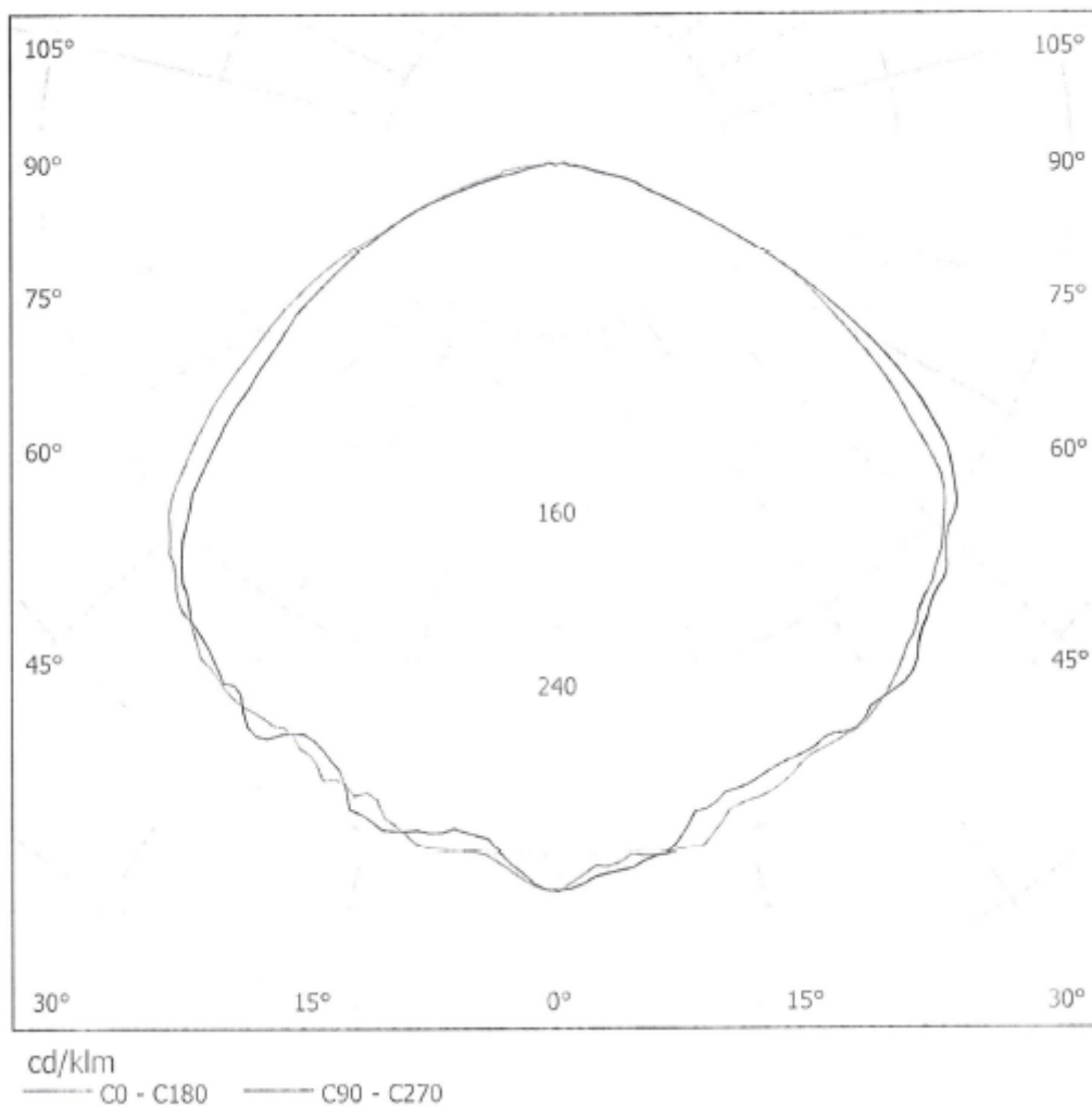
Кривые распределения силы света в 2 плоскостях светодиодного светильника ДСП47-45 Б С
