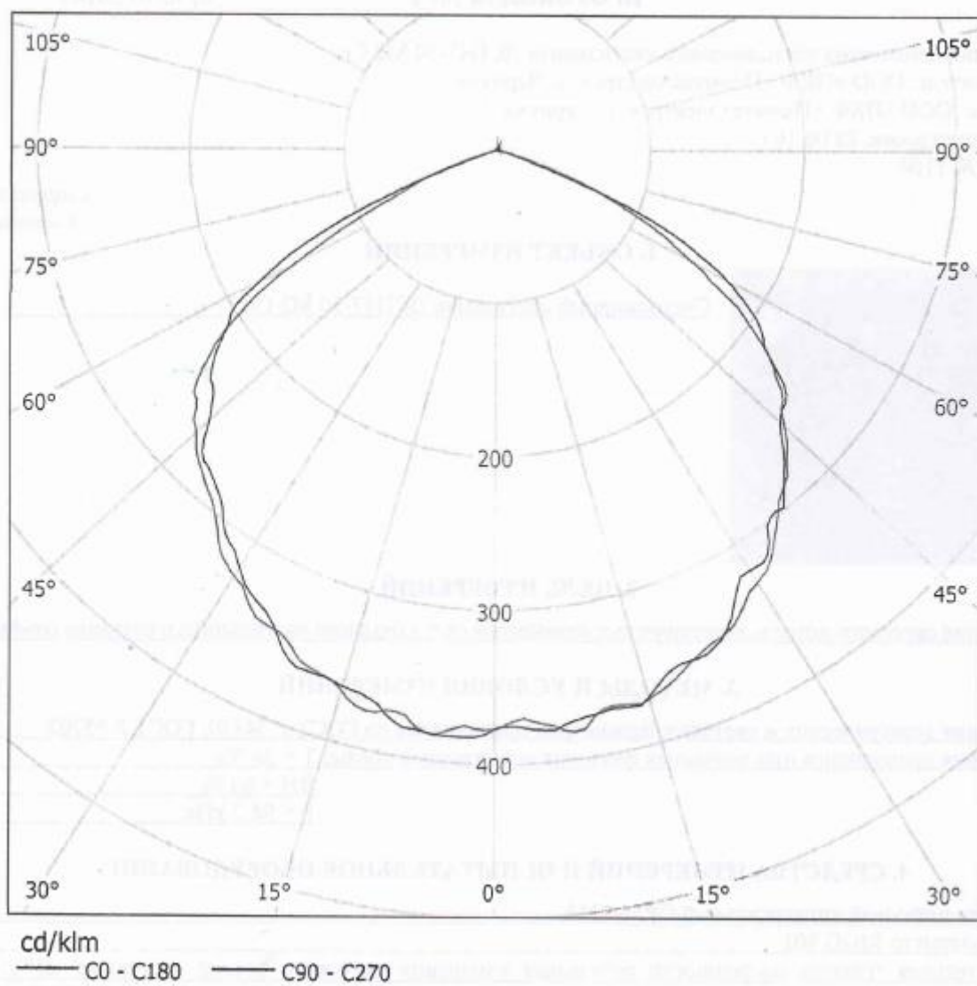
Кривые распределения силы света в 2 плоскостях светодиодного светильника ДСП47-30 М2 Сп
