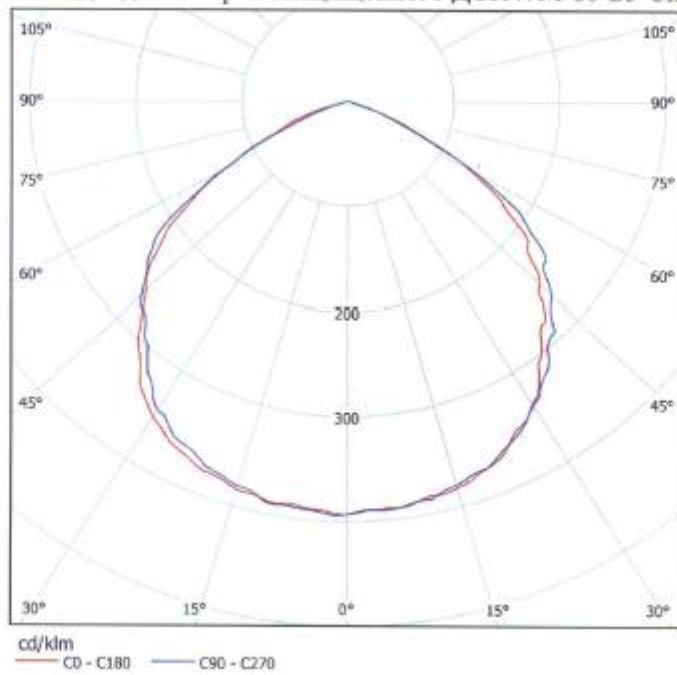
Кривые распределения силы света в 2 плоскостях светильника светодиодного взрывозащищённого ДСП47М-80-Б3-Сп, УХЛ1, IP67
