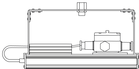
комбинированный подвес (натрубу G3/4")
