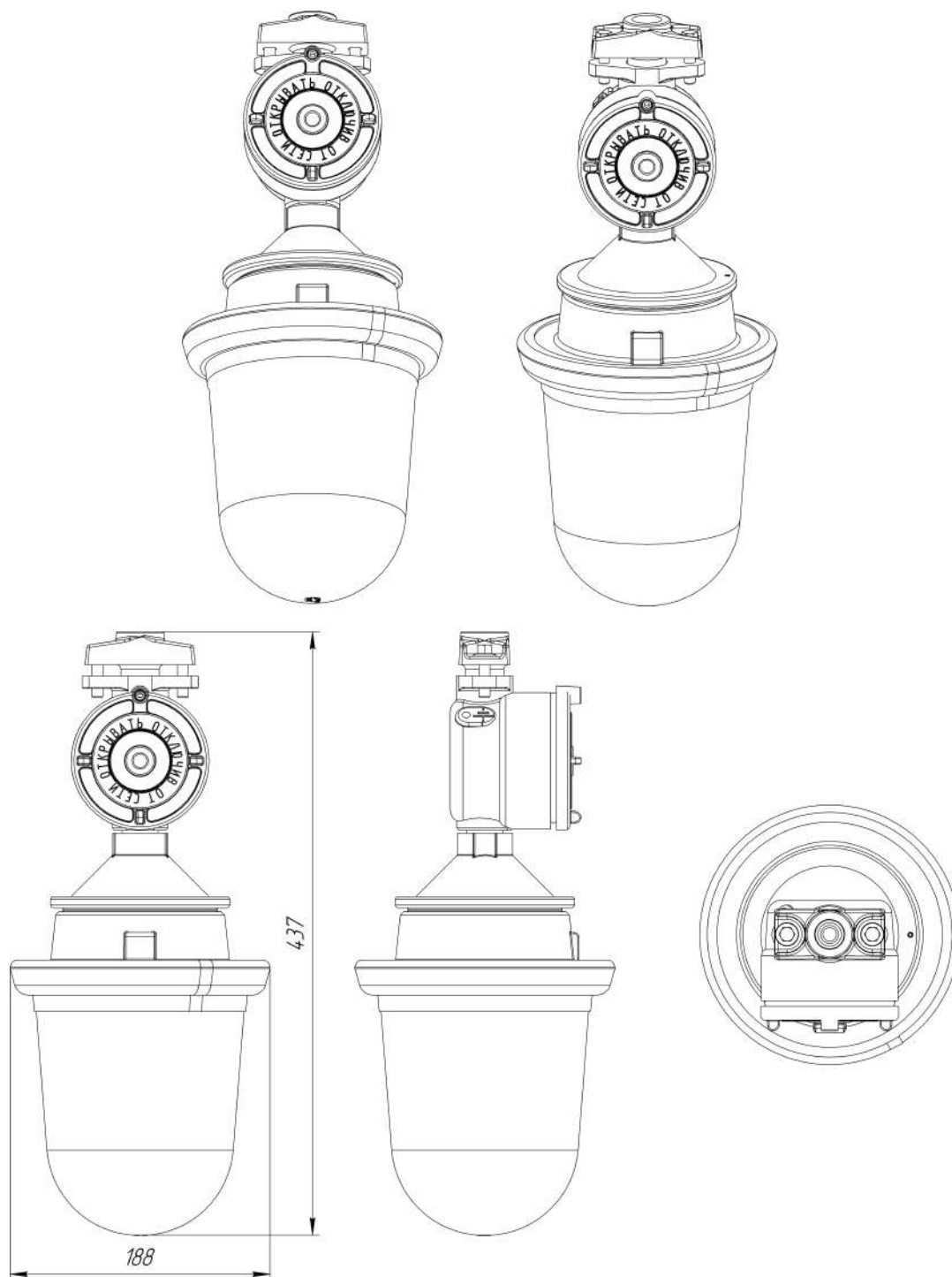
Габаритный чертеж ВЗГ-200-М2 (ЛОН)
