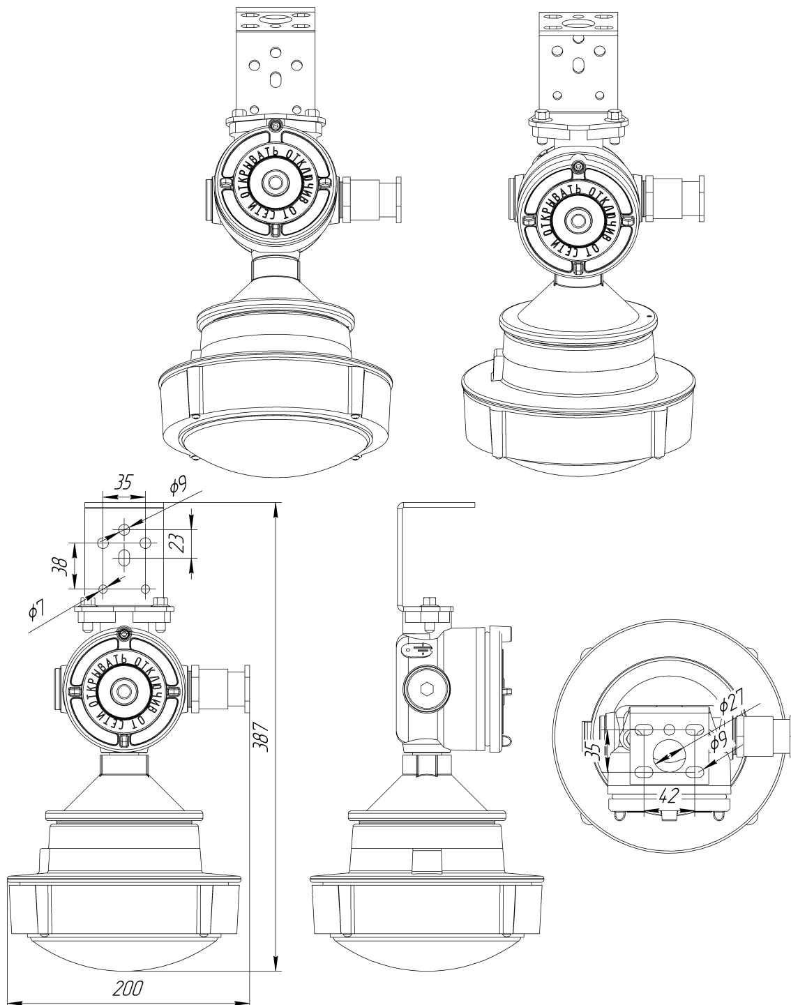
Габаритный чертеж ВЗГ-200ДМ-20-М3-Сп
