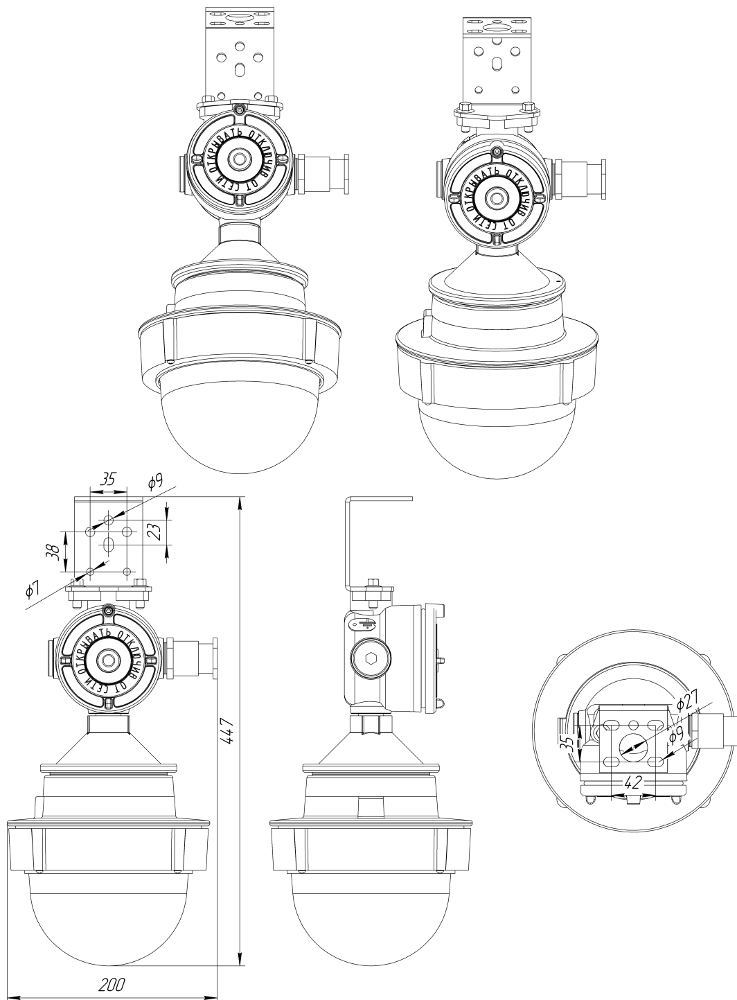
Габаритный чертеж ВЗГ-200ДМ-25-М3-Су-НВ
