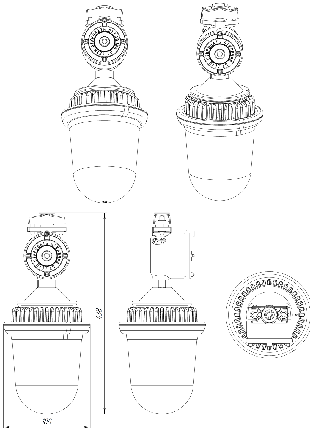
Габаритный чертеж ВЗГ-200Дн-15-М2
