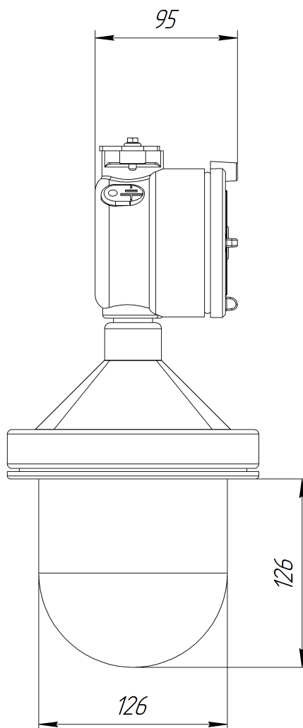
Габаритный чертеж ВЗГ-200н-1-15-М2-НВ
