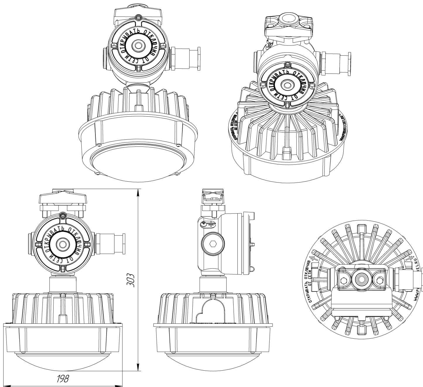
Габаритный чертеж ДСП48-15-М2-Сп-02-Тр
