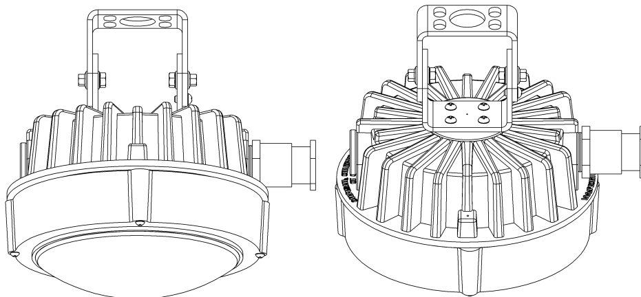
Габаритный чертеж ДСП48-15-Сп-02-НП-НВ
