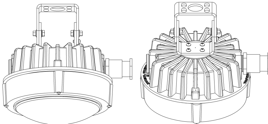
Габаритный чертеж ДСП48-15-СП-02-НП
