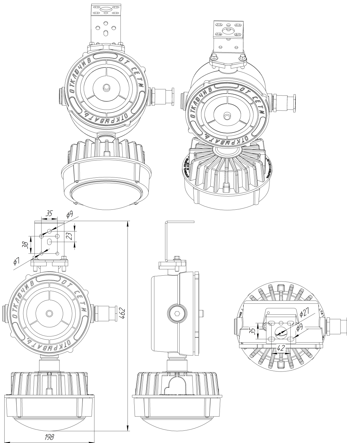
Габаритный чертеж ДСП48-20-Б3-Сп-02-НВ
