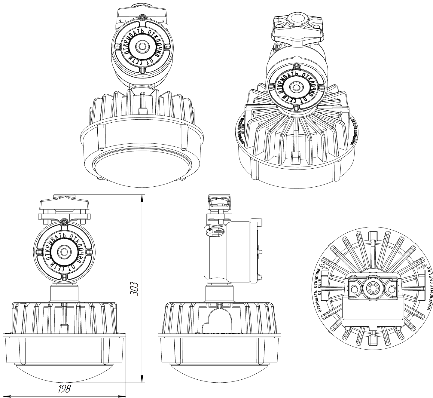
Габаритный чертеж ДСП48-20-М2-Сп-02-НВ
