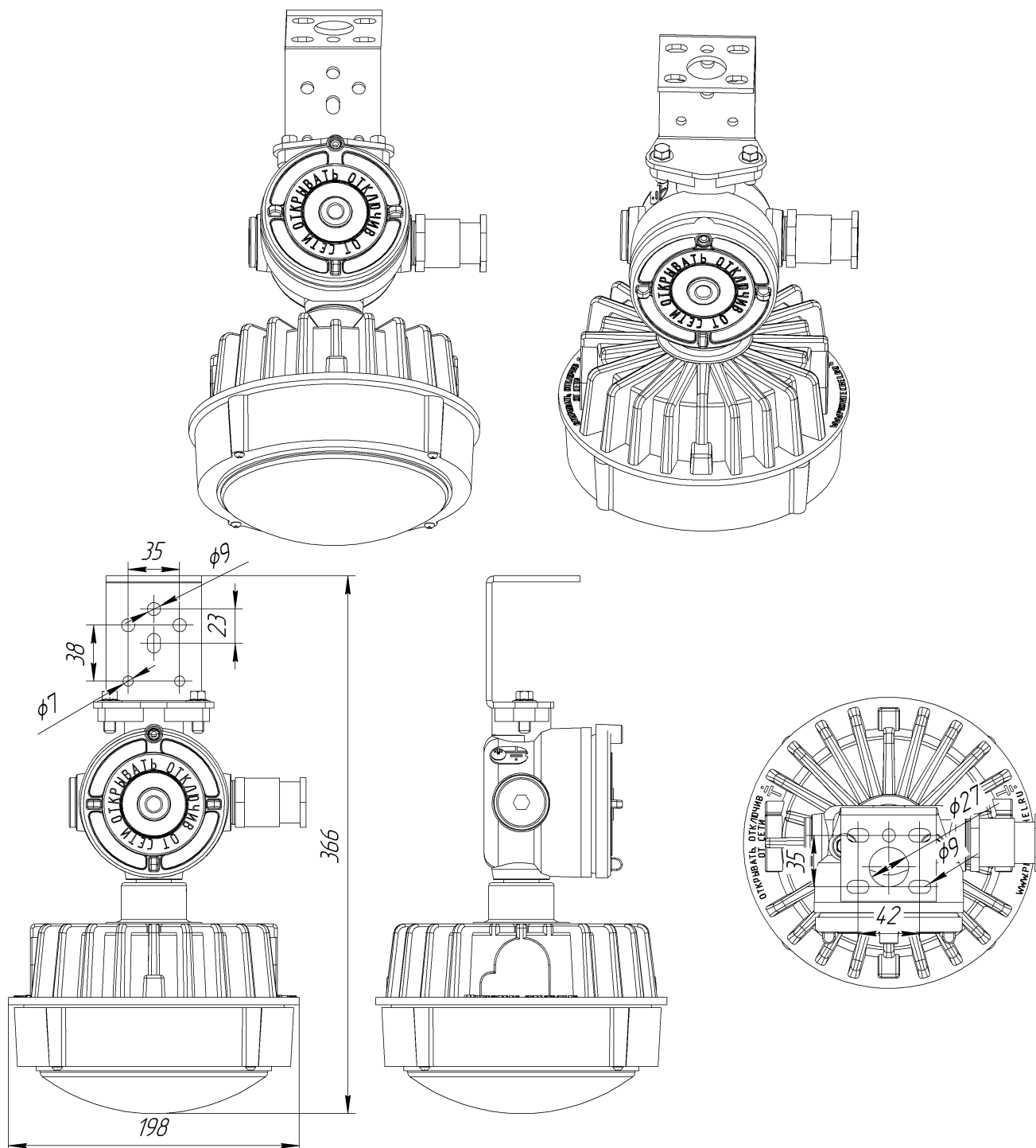
Габаритный чертеж ДСП48-20-М3-Сп-02-Тр
