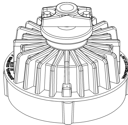
Габаритный чертеж ДСП48-20-Сп-02-НВ
