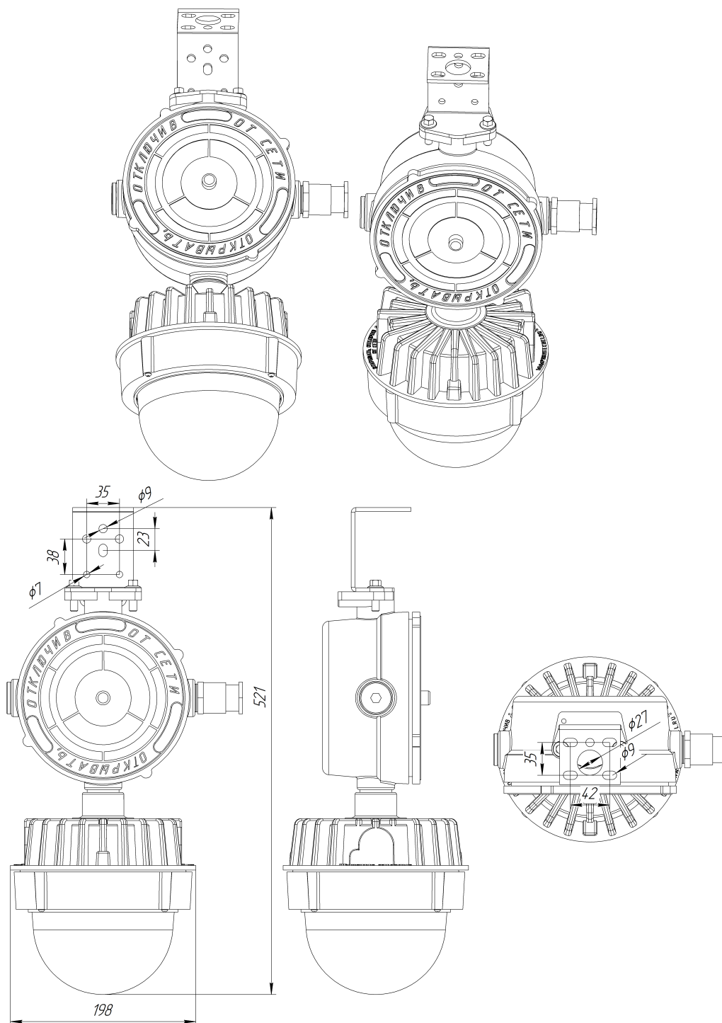
Габаритный чертеж ДСП48-25-Б3-Су-02
