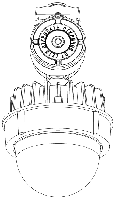
Габаритный чертеж ДСП48-25-М2-Су-02
