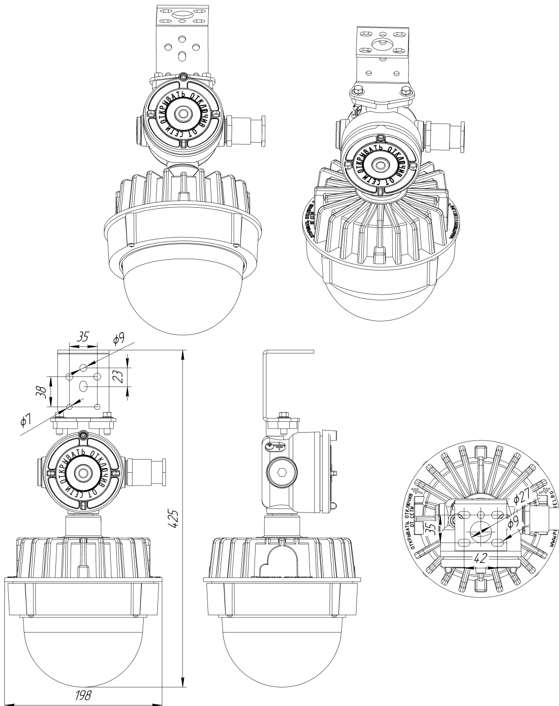
Габаритный чертеж ДСП48-25-М3-Су-02-НВ
