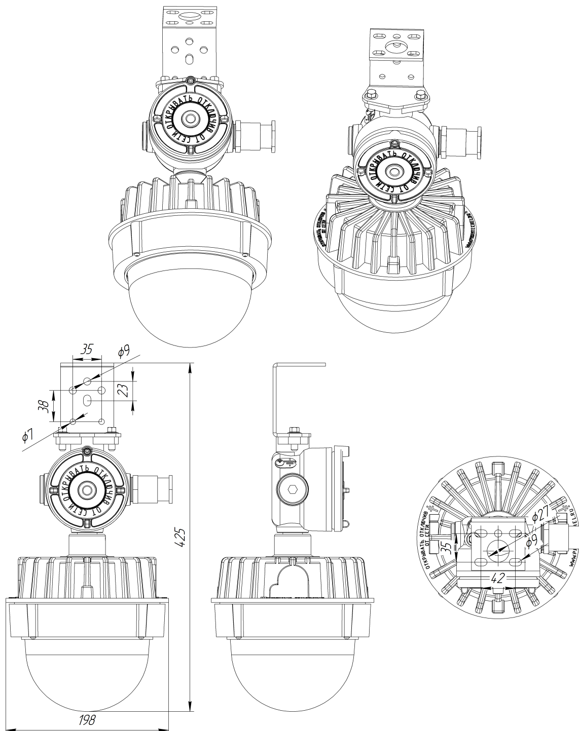
Габаритный чертеж ДСП48-25-М3-Су-02-Тр-НВ
