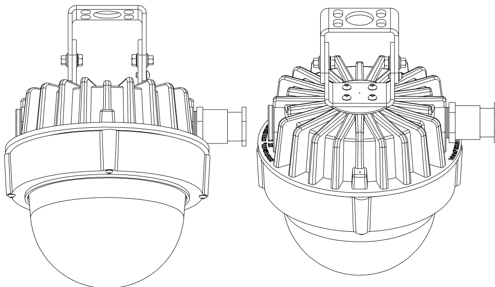
Габаритный чертеж ДСП48-25-Су-02-НП-НВ
