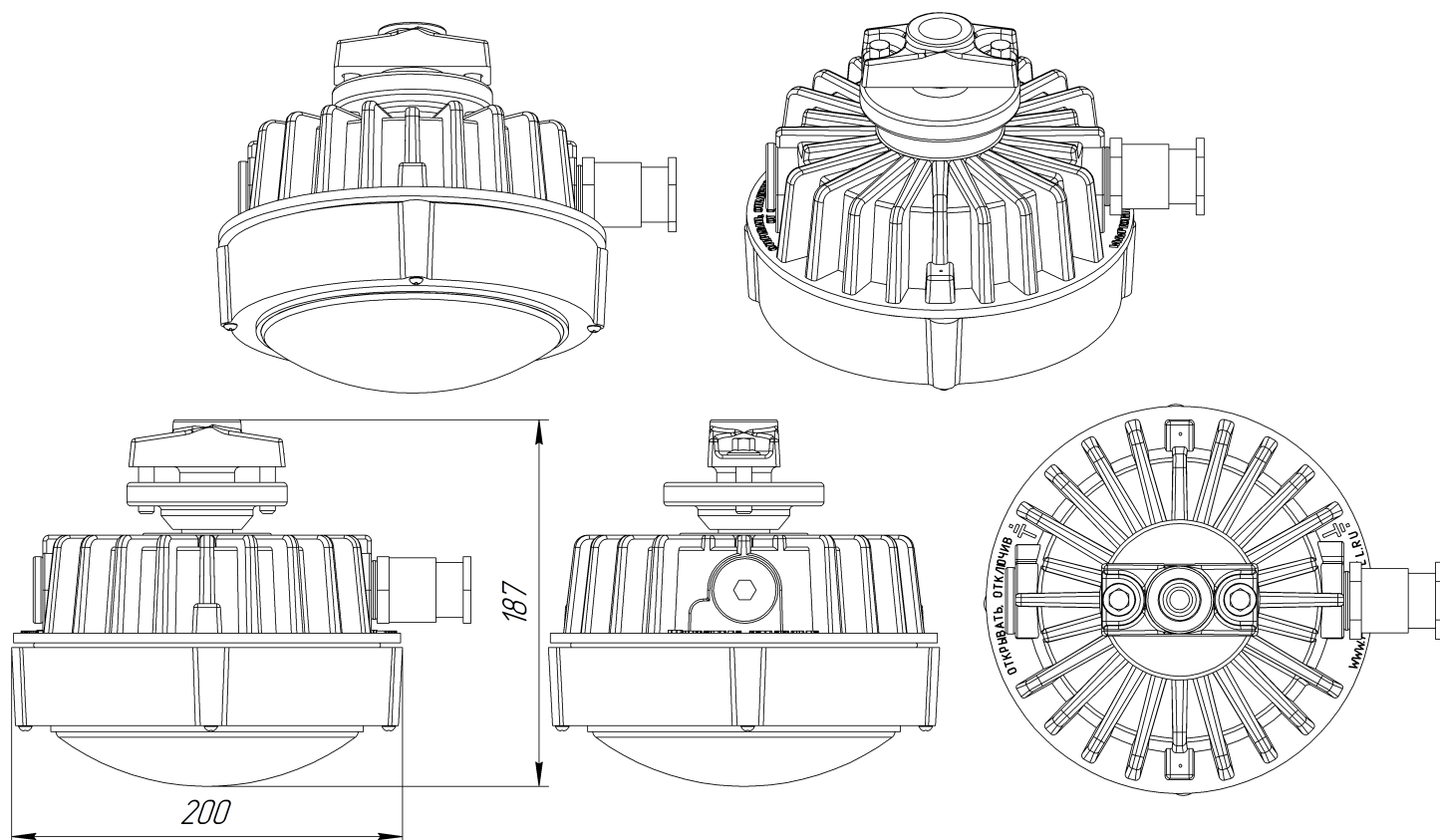
Габаритный чертеж ДСП48-30-Сп-02-Тр-НВ
