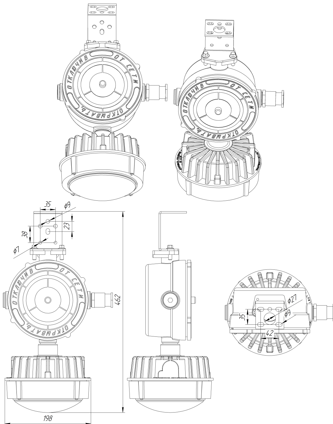
Габаритный чертеж ДСП48-40-Б3-Сп-02-НВ
