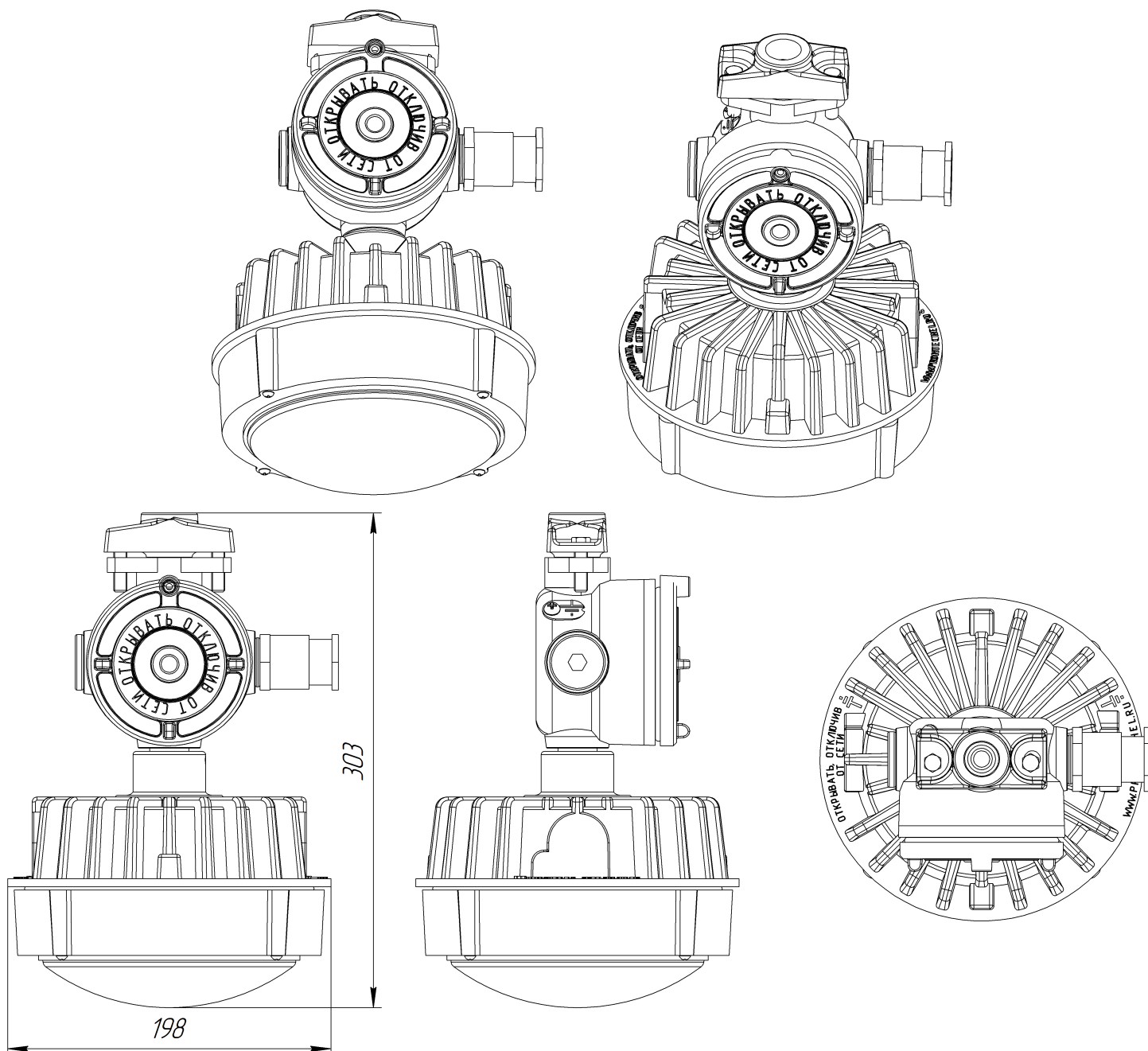
Габаритный чертеж ДСП48-40-М2-СП-02-ТР-НВ
