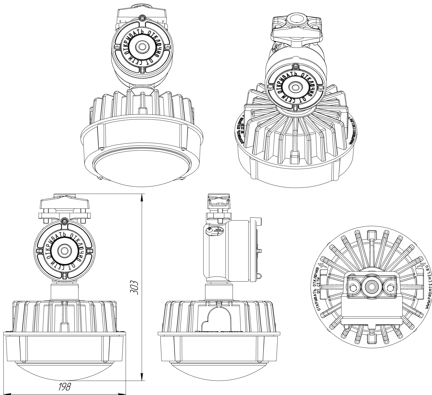
Габаритный чертеж ДСП48-40-М2-Сп-02
