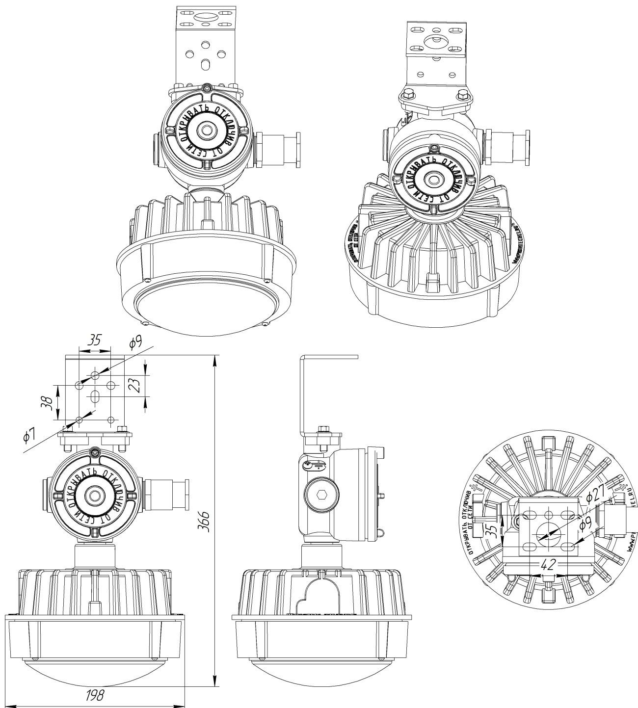
Габаритный чертеж ДСП48-40-М3-СП-02-ТР-НВ
