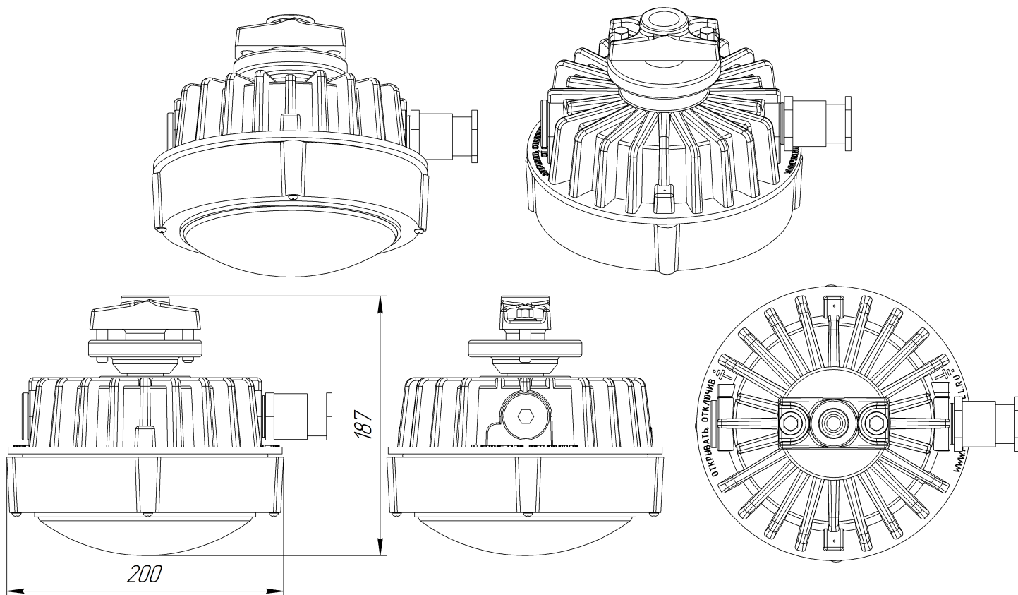
Габаритный чертеж ДСП48-40-Сп-02-Тр
