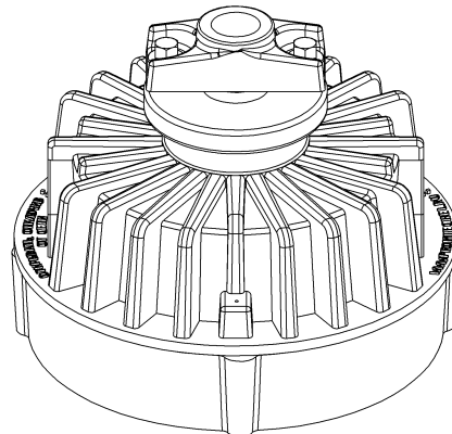
Габаритный чертеж ДСП48-40-Сп-02
