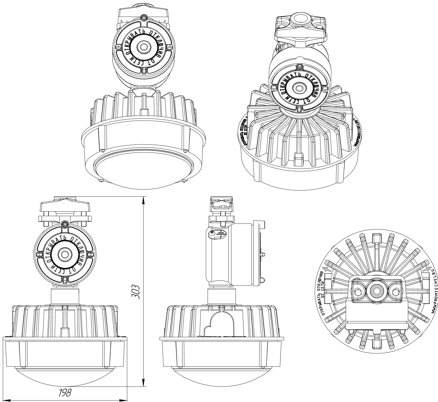
Габаритный чертеж ДСП48-50-М2-Сп-02-НВ
