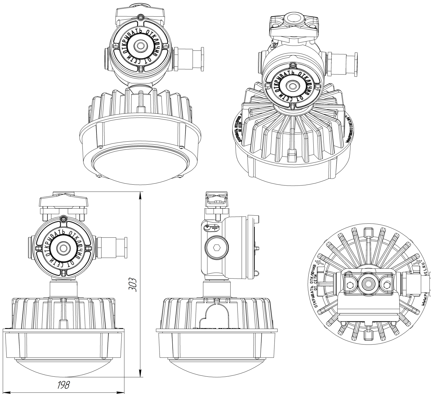
Габаритный чертеж ДСП48-50-М2-СП-02-Тр
