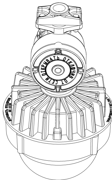
Габаритный чертеж ДСП48-50-М2-Су-02-Тр
