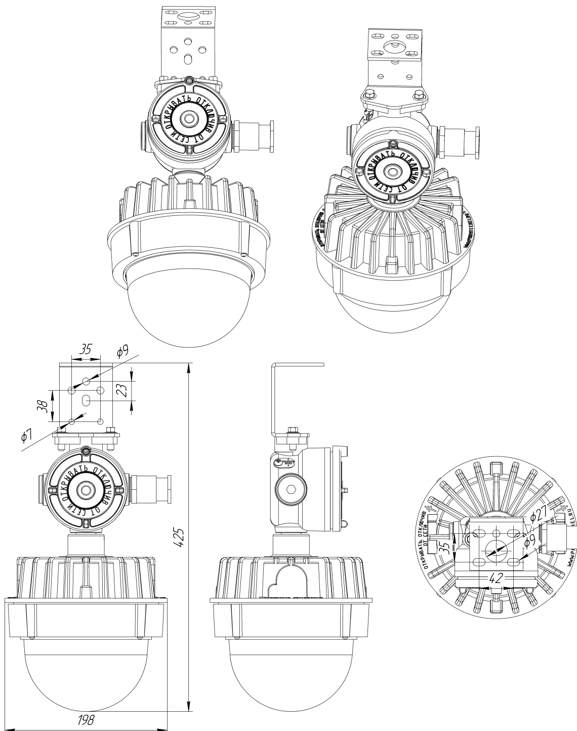
Габаритный чертеж ДСП48-50-М3-Су-02-Тр-НВ
