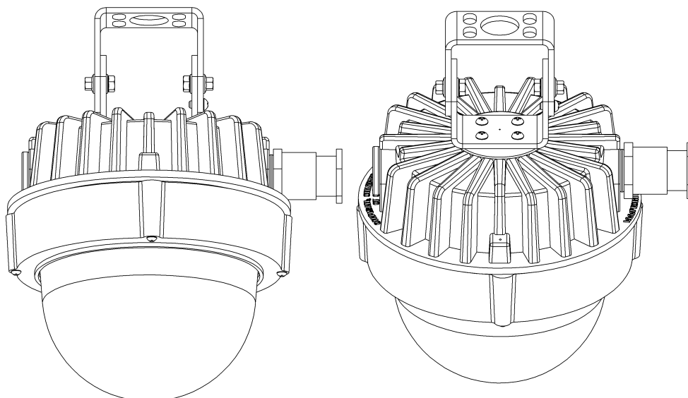
Габаритный чертеж ДСП48-50-Су-02-НП
