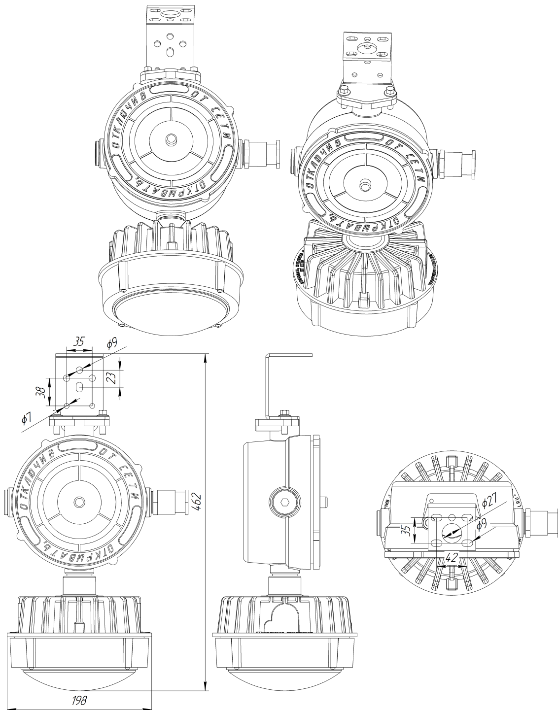
Габаритный чертеж ДСП48-80-БЗ-Сп-02
