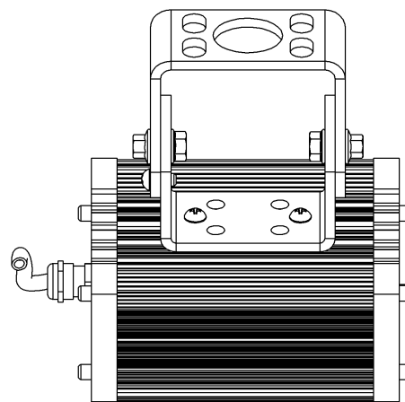
Габаритный чертеж ДСП52-15-000
