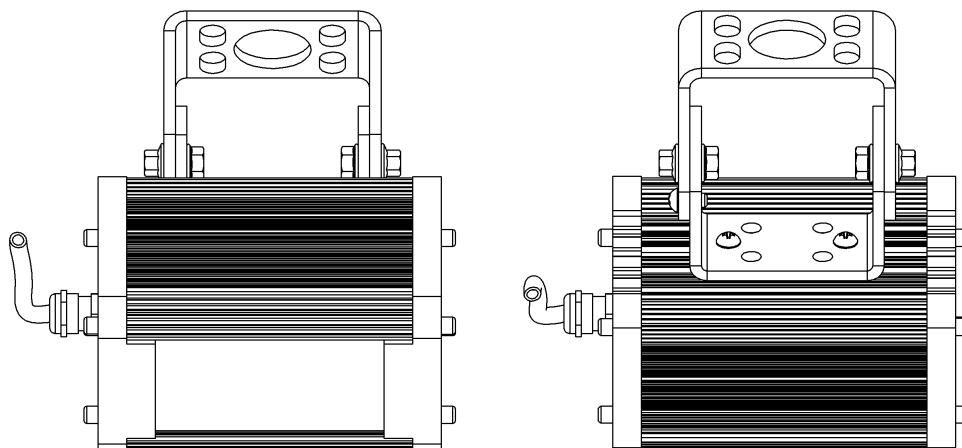
Габаритный чертеж ДСП52-15н-000
