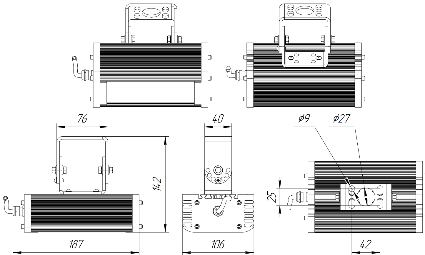
Габаритный чертеж ДСП52-20н-000
