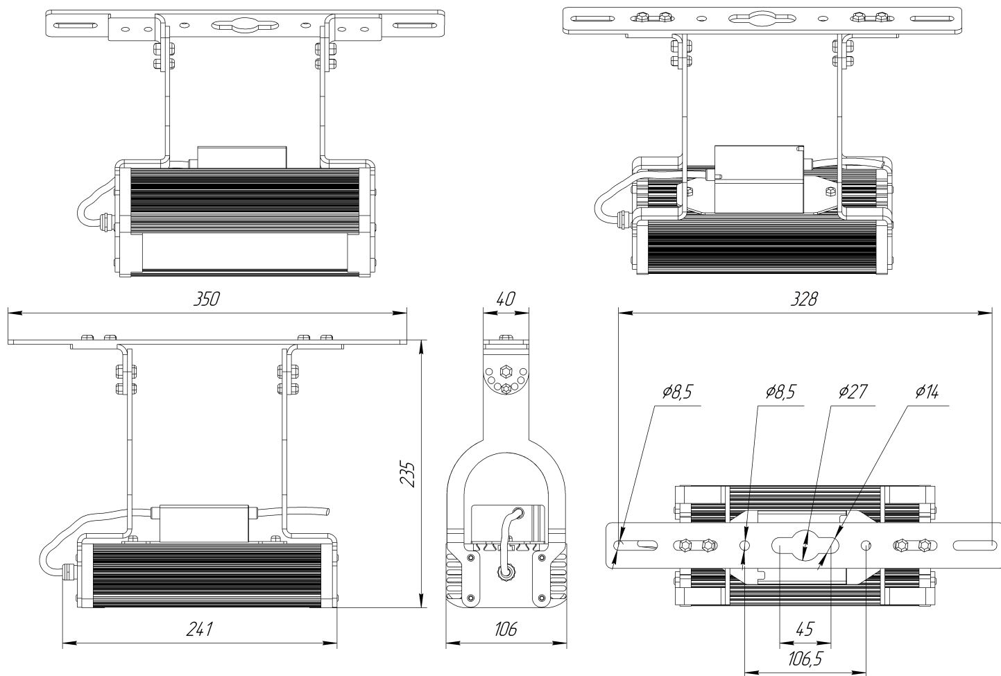
Габаритный чертеж ДСП52-30-000
