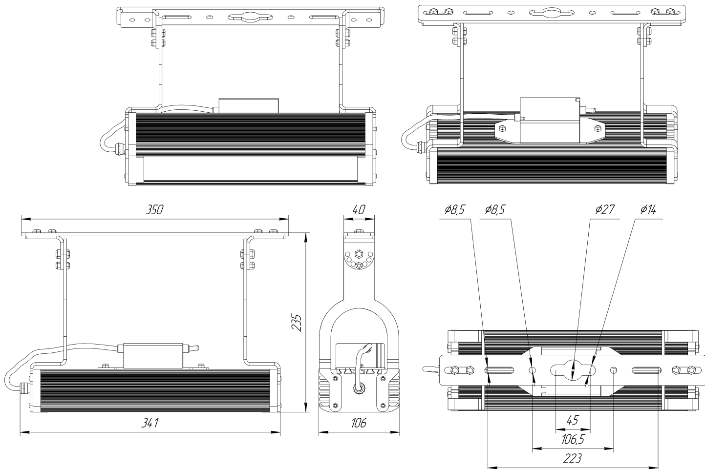
Габаритный чертеж ДСП52-45Н-000
