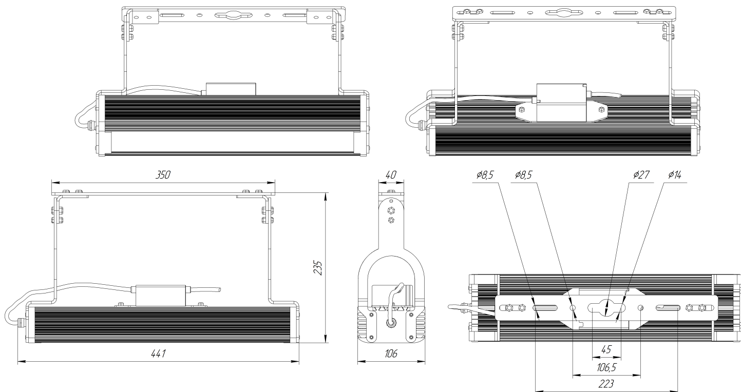
Габаритный чертеж ДСП52-60н-000
