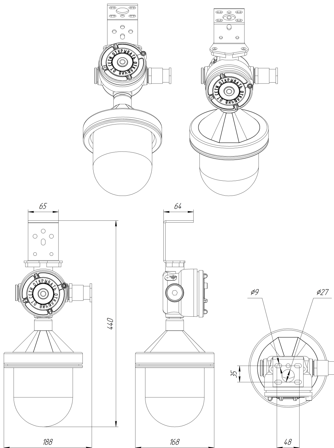
Габаритный чертеж ВЗГ-200н-2-30-МЗ-НВ
